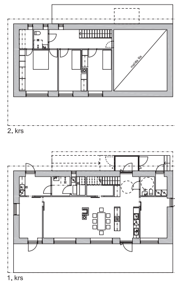
Kuva 4: Esimerkki pohjaratkaisusta, jossa tilat ja pääosa ikkuna-pinta-alasta on suunnattu etelään.
