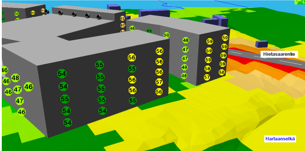
Kuva 1. Hartaanselän puoleiselle julkisivulle kohdistuvat päiväajan keskiäänitasot (LAeq,7-22)
