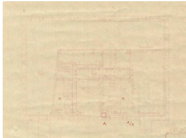
Kuva 20. Alkuperäinen rakennuslupapiirustus, kellarin pohjapiirustus.
