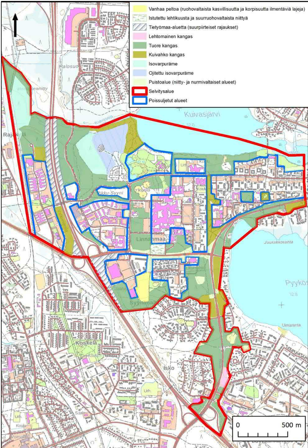
Kuva 27. Selvitysalueen kasvillisuustyyppit.
