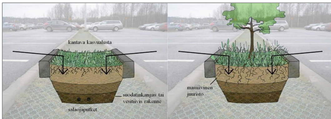
Kuva 13. Periaatteellinen kuva hulevesiä viivyttävästä ja suodattavasta viherpainanteesta. Kuva: Vantaan kaupunki, Porttipuiston pysäköintialueen rakennussuunnitelma.
