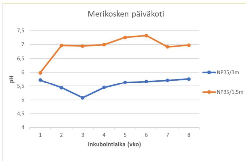
Kuva 2 Merikosken päiväkotii sulfaattimaanäytteiden pH:n muutos inkuboinnin aikana.
