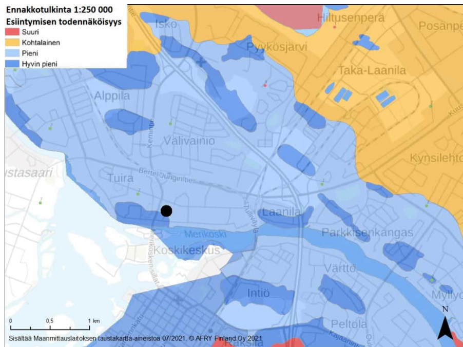
Kuva 1 GTK:n ennakkotulkinta happamien sulfaattimaiden esiintymisen todennäköisyydestä Oulun alueella. Merikosken päiväkodin tutkimusalueen sijainti on merkitty mustalla pisteellä. (Geologian tutkimuskeskus 2020).
