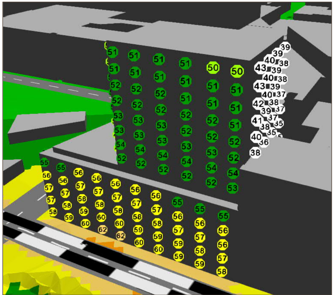
Kuva 6. Tie- ja raitioliikenteen aiheuttamat suurimmat keskiäänitasot julkisivuittain yöaikaan
