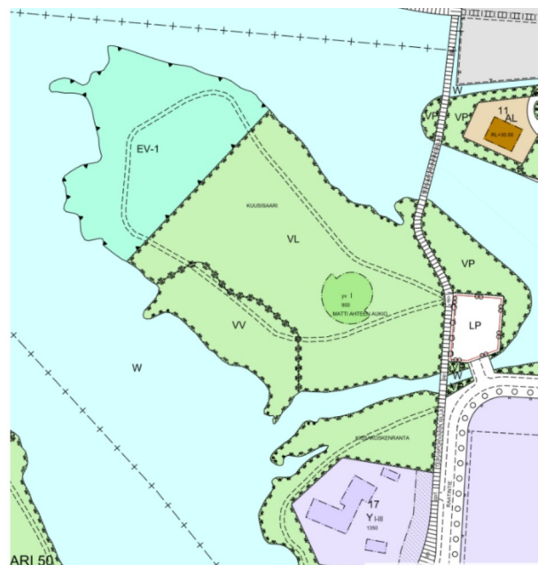
Kuva 2. Ote ajantasa-asetuksesta
