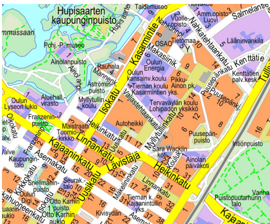
Kuva 1. Suunnittelualue osakartalla
