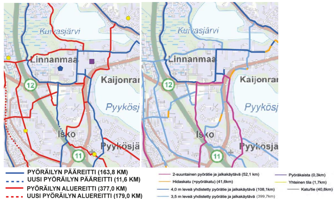
Kuva 10. Suunnittelualan pyöräteiden luokittelu ja kehittämislähtöisen tavoitetilan pyöräväylien teknisestä ratkaisusta (lähde: Oulun seudun pyöräilyn pääreitissuunnitelma 2030, Ramboll Oy).
