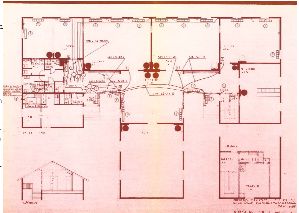
Nokkalan ala-asteen sähkölämmityksen johdotuspiirustus 8.2.1988, Oulun Tilakeskuksen arkistosta löytynyt piirustus.
