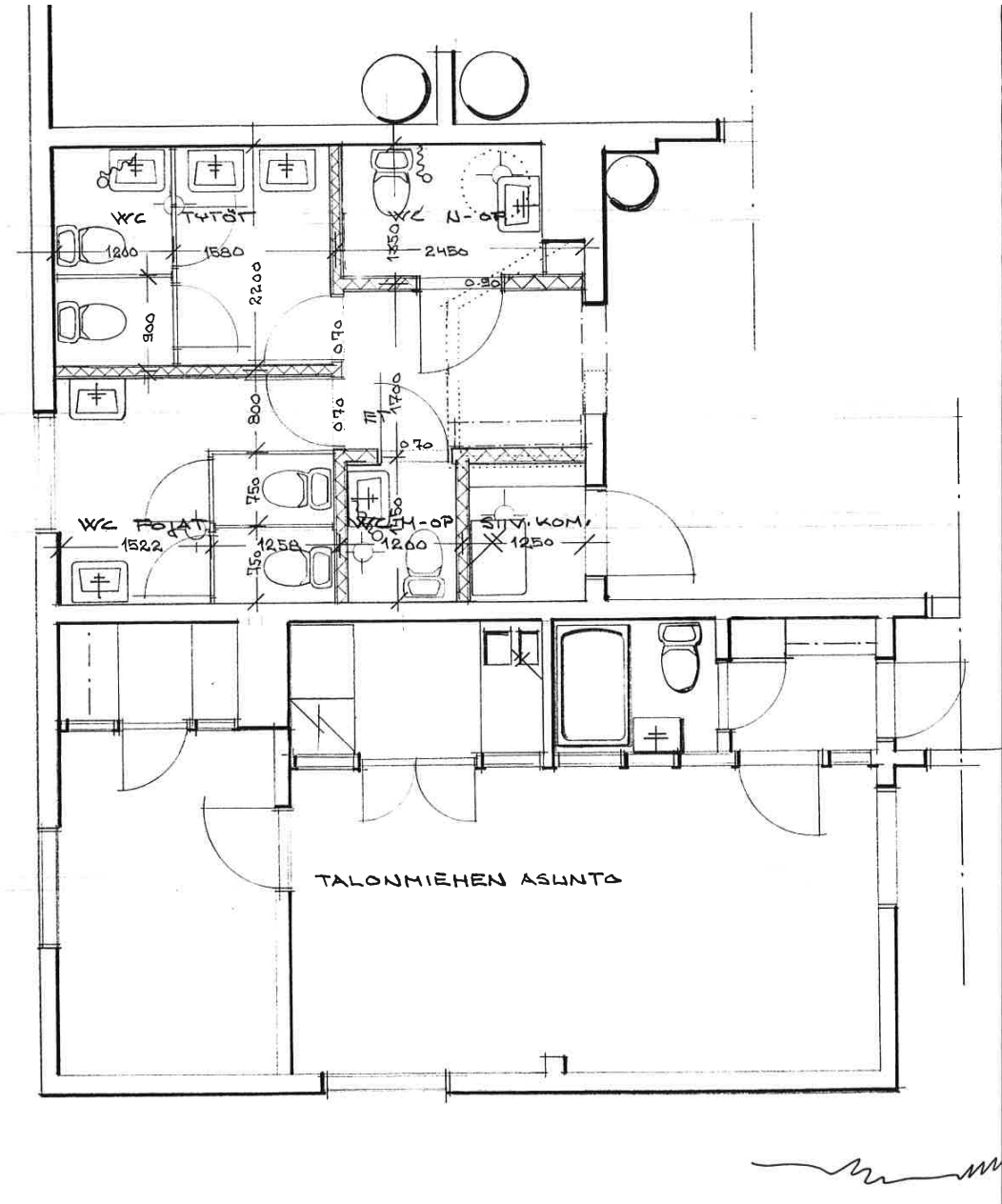
Nokkalan ala-asteen sisäWCt 14.6.1985, Oulun Tilakeskuksen arkistosta löytynyt piirustus.
