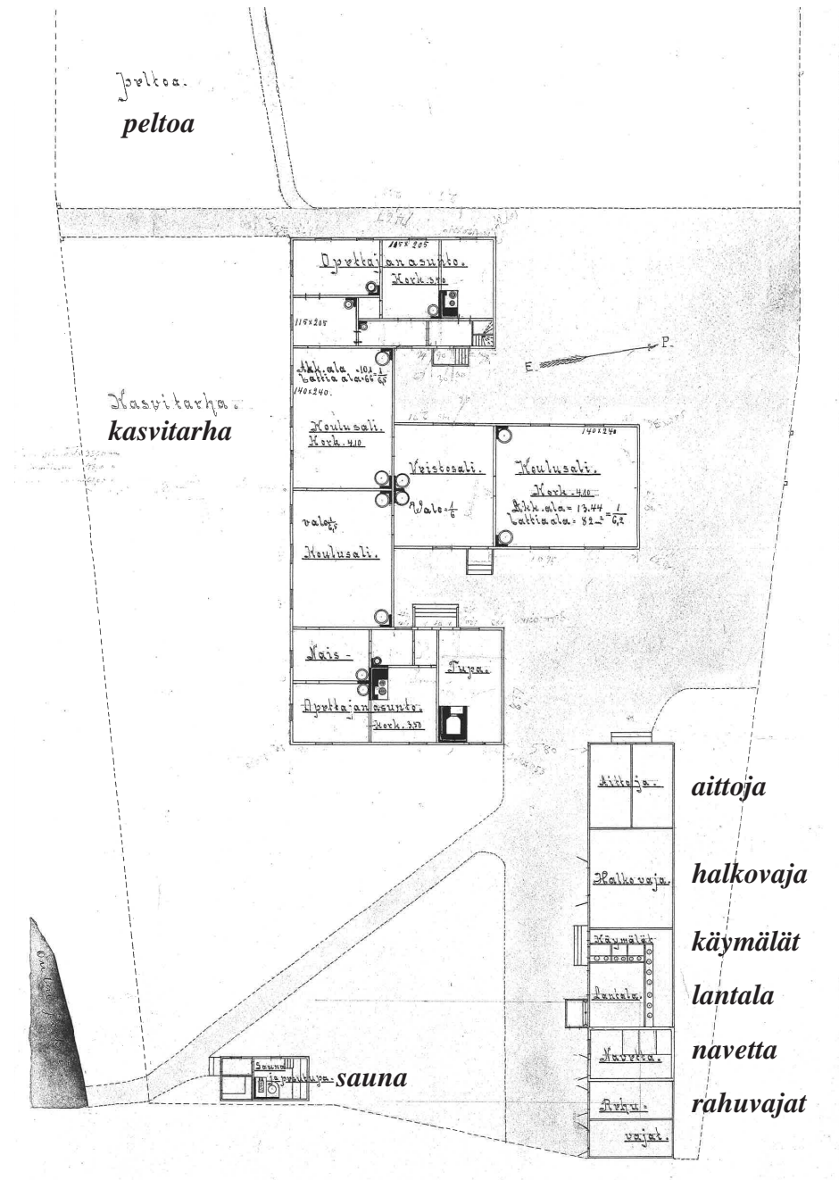
Laanilan kansakoulun asema- ja pohjapiirustus vuodelta 1910. Kansakoulun tarkempi pohjapiirros sivulla 11. Oulun Tilakeskuksen arkisto.
