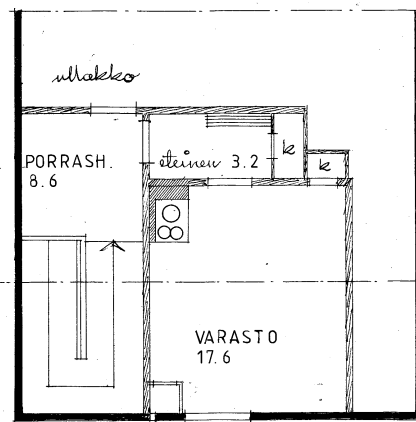
PIIRUSTUS TARKISTETTU 10.12.1979 (TL) OULUN KAUP. RAKENNUS-TOIMISTO 26.4.1945
