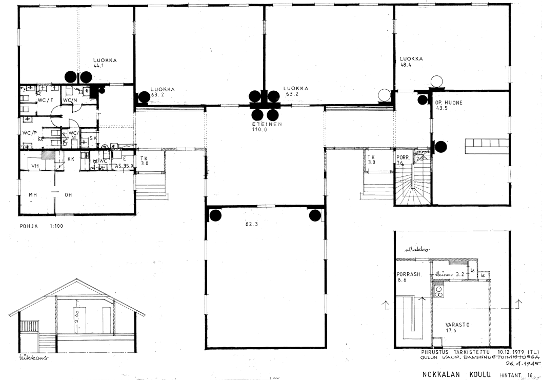
Laanilan kansakoulun muutostyö 1945. Piirustuksessa myös täydennyksiä vuodelta 1979. Oulun Tilakeskuksen arkisto
