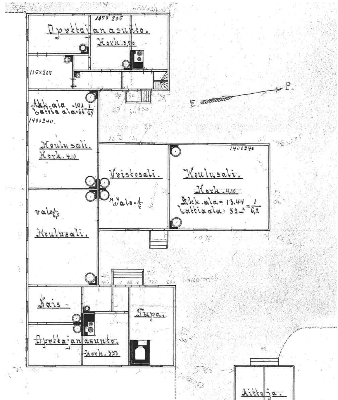
Laanilan kansakoulun pohjapiirustus vuodelta 1910. Oulun Tilakeskuksen arkisto.
